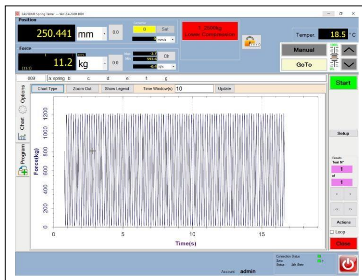
Graphique Force / Temps
