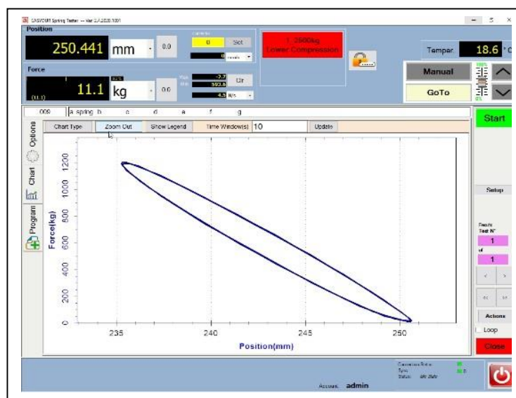
Graphique Force / Position
