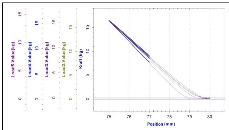
Graphique multicanal Force / Position
